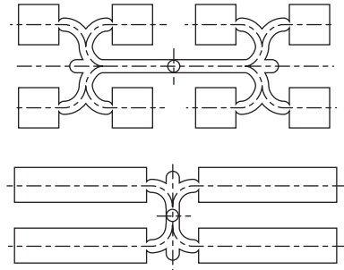
スプルーから各ゲートまでの距離を等しくしてバランスをとる
